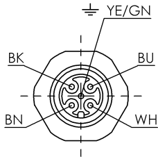
Вид в сторону штекера
