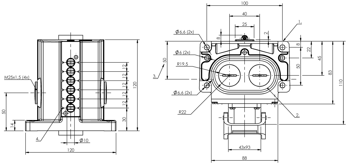
1) Опорная кромка, 2) Уплотнительное кольцо, 3) Кабельный ввод, 4) Марк. Безопасн. точка переключения
