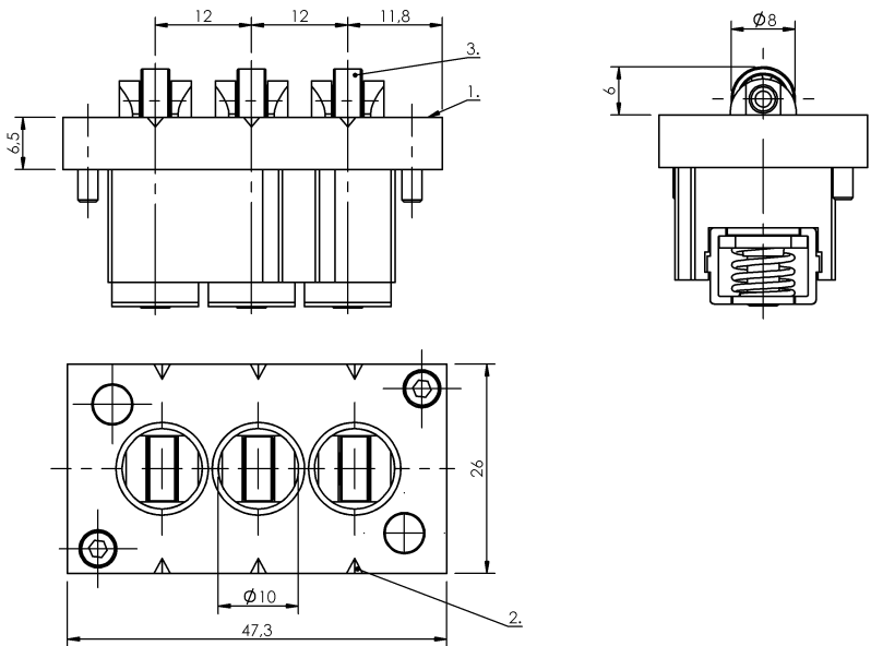
1) Опорная кромка, 2) Марк. Безопасн. точка переключения, 3) 1-я точка переключения
