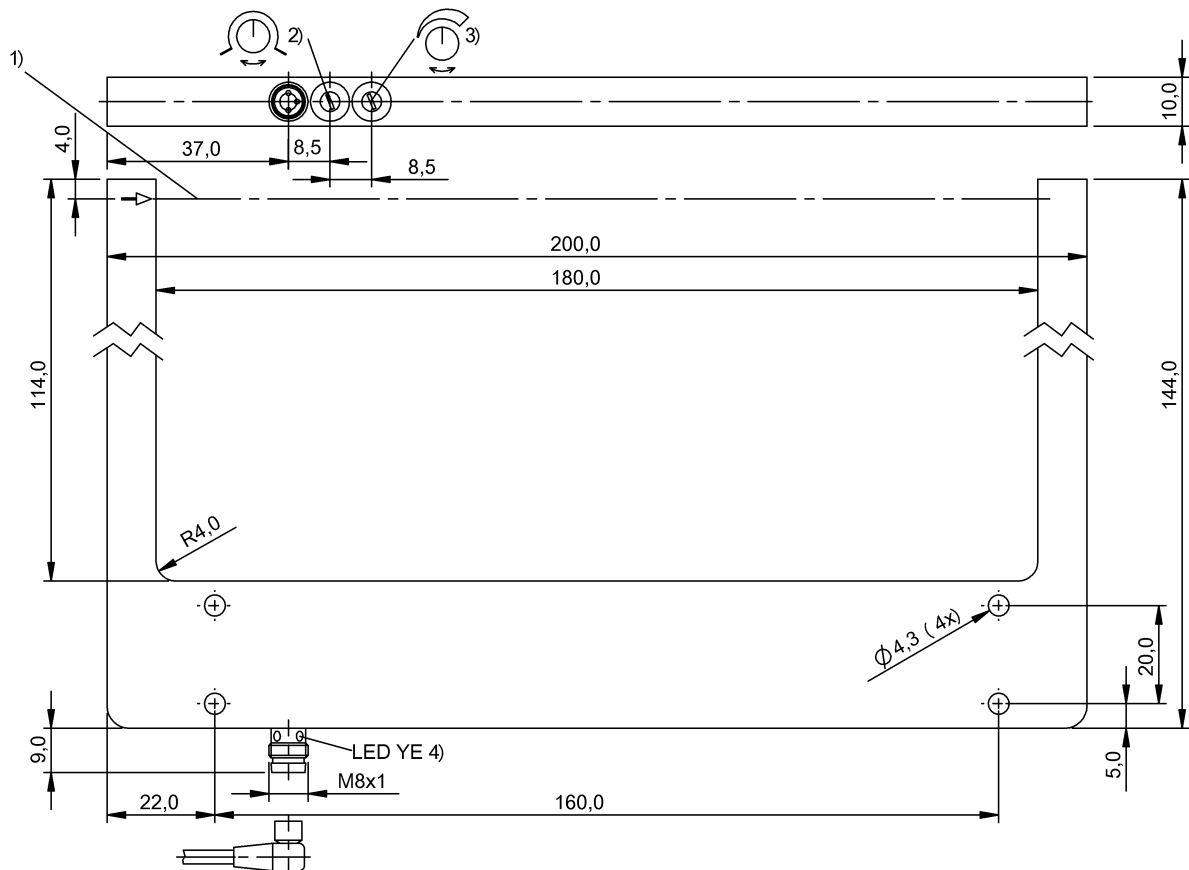
1) Eixo ótico, 2) Sensibilidade, 3) Comutação claro/escuro, 4) Função de saída
